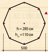
SAVOTTA SA-20
